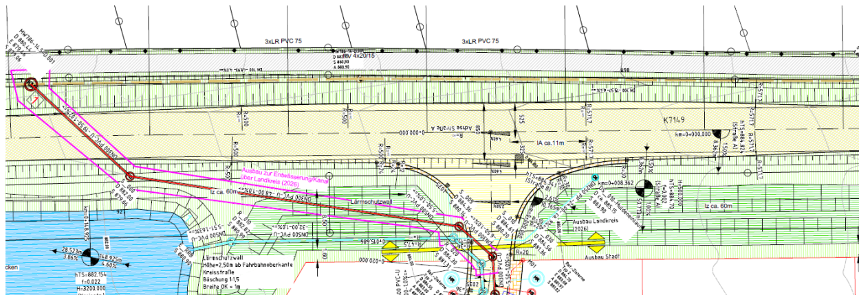
Linksabbieger Kreisstraße 7149 - Grund/Hülbenwiesen
