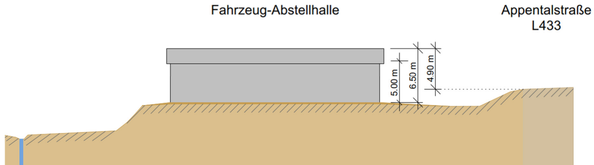
Abbildung 2: Darstellung des geplanten Vorhabens im Schnitt
